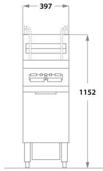
Frontansicht
