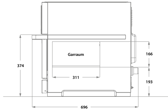
Seitenansicht
