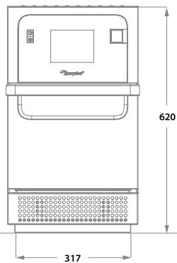
Frontansicht
