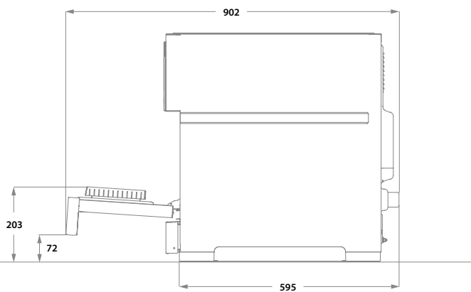
Seitenansicht
